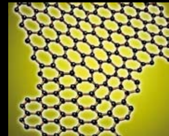
Grafeenstructuur
